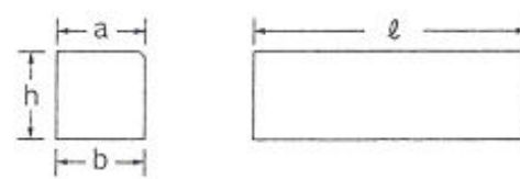
(地先境界ブロック)
