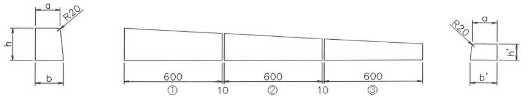
三段乗入れ左 (右)
