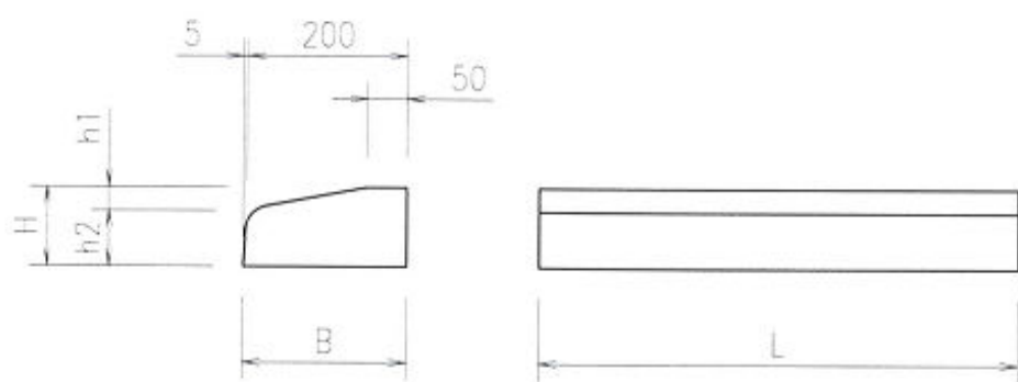
乗入タイプ・車両乗入部 セミフラットタイプ
