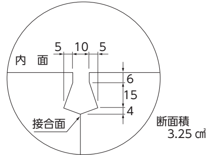
目地部詳細図
